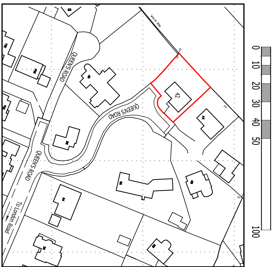
Site Plan 1:1250
