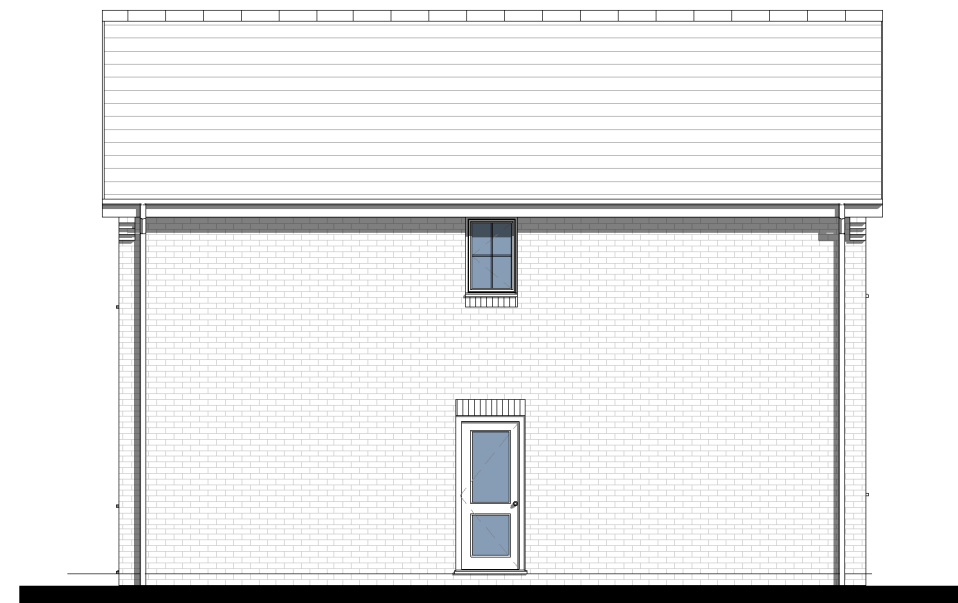
3 Rear 1 : 100
