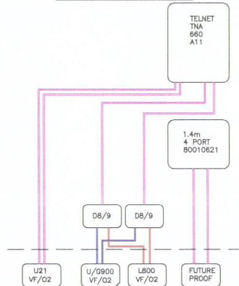
ANTENNA SCHEMATIC N.T.S.
