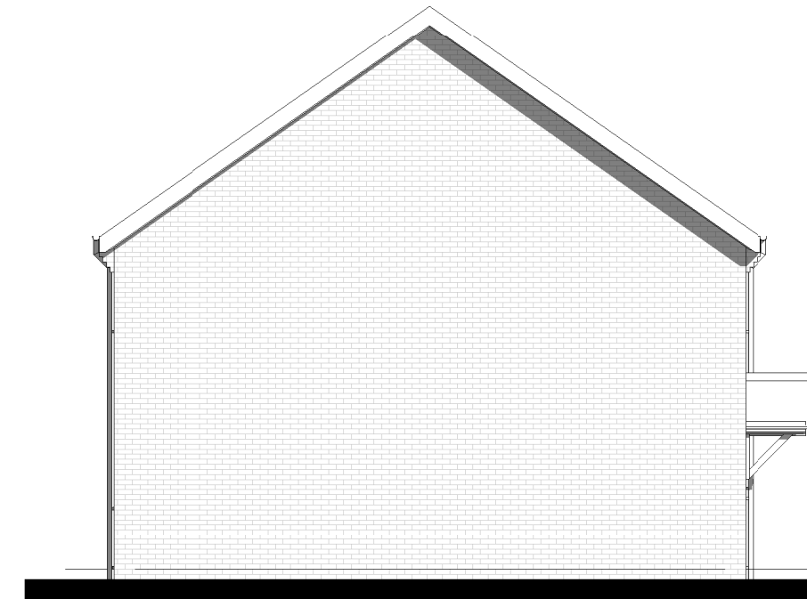
4 Gable 2 1 : 100
