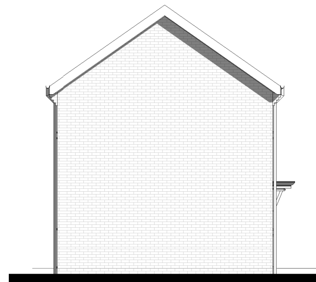
4 Gable 2 1 : 100
