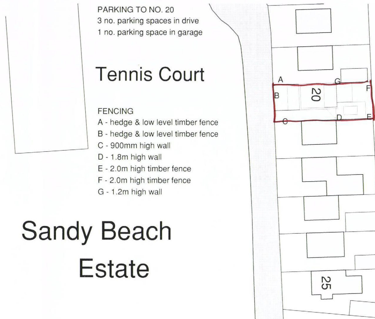
Site Plan 1:500
