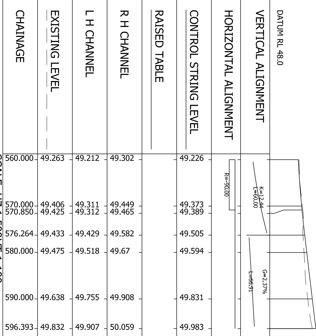
LONGITUDINAL SECTION - MC02
