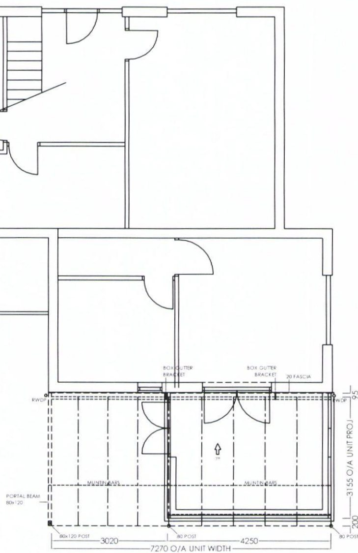
PROPSOED PLAN
