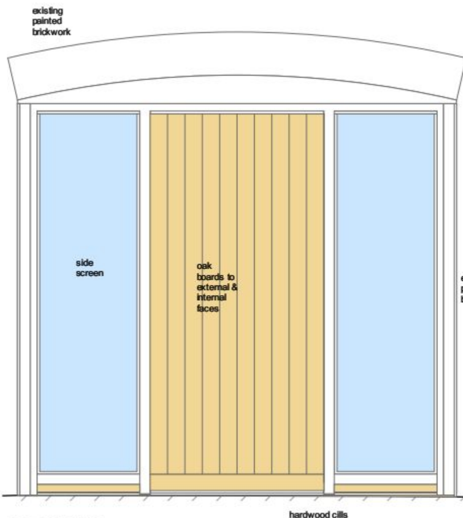
ELEVATION
