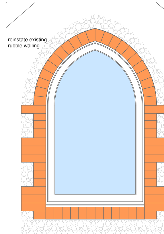
ELEVATION
