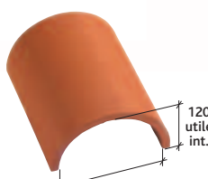
Faîtière 1/2 ronde sans emboîtement (3 au ml) Réf. 718 *
