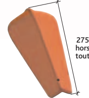
About d'arêtier angulaire sans emboîtement Réf. 864 *
