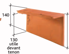
Rive individuelle droite (1) (5 à 6 au ml) Réf. 500.45 *
