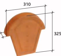
Fronton pour faîtière 1/2 ronde à recouvrement Réf. 807 *
