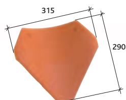
Noue à 45° (1) Réf. 500.146 *
