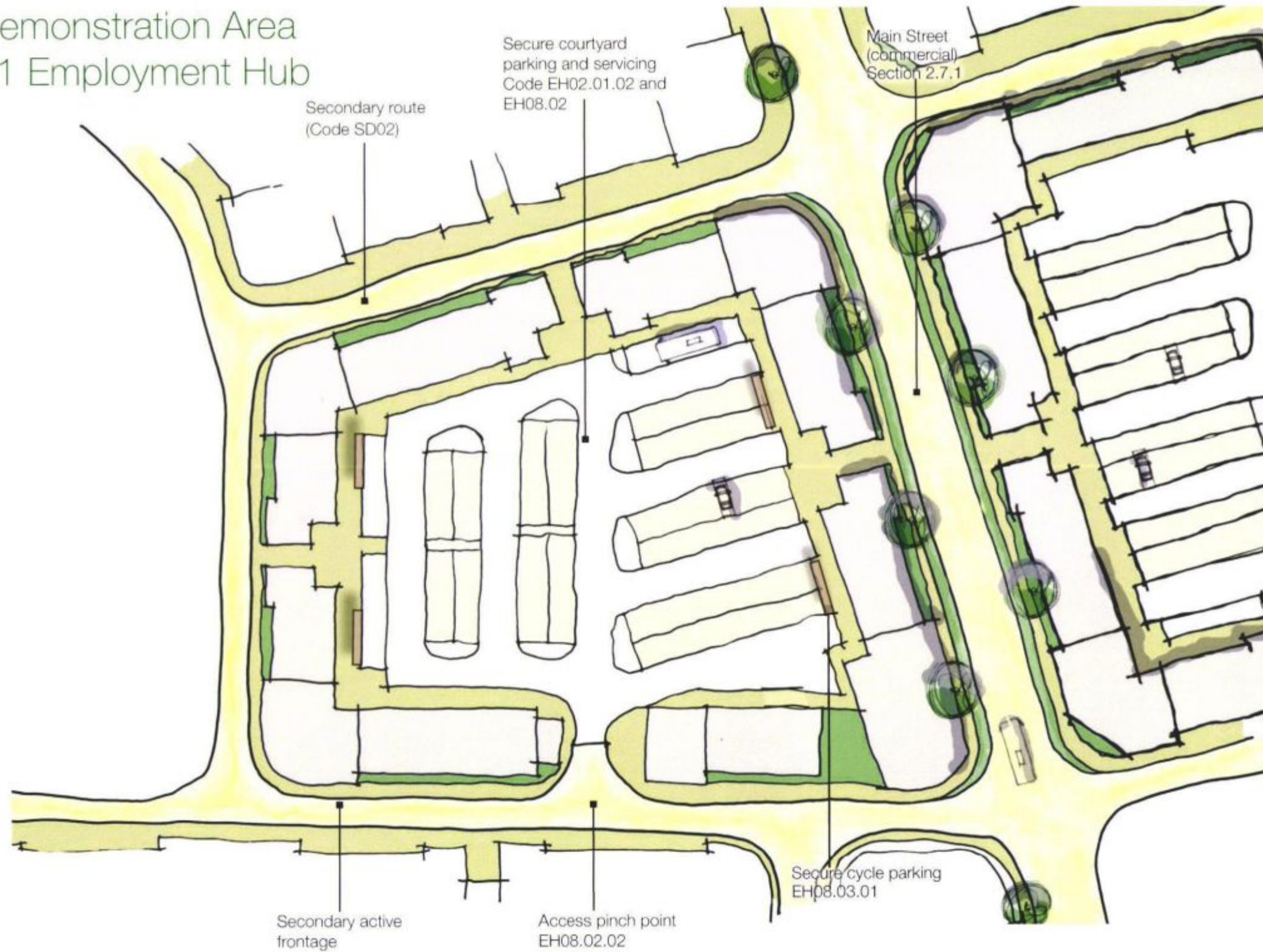
E1 Plan
