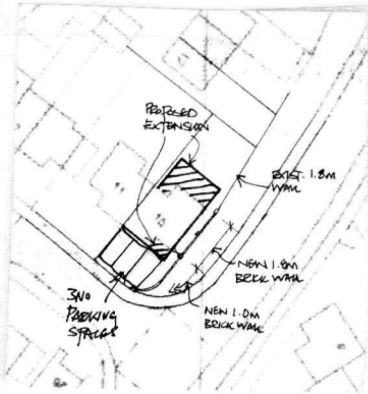
SITE PLAN 1:500
