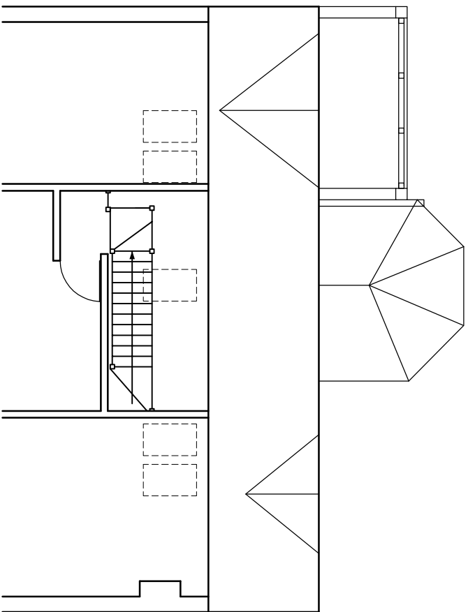
Loft plan 1:100
