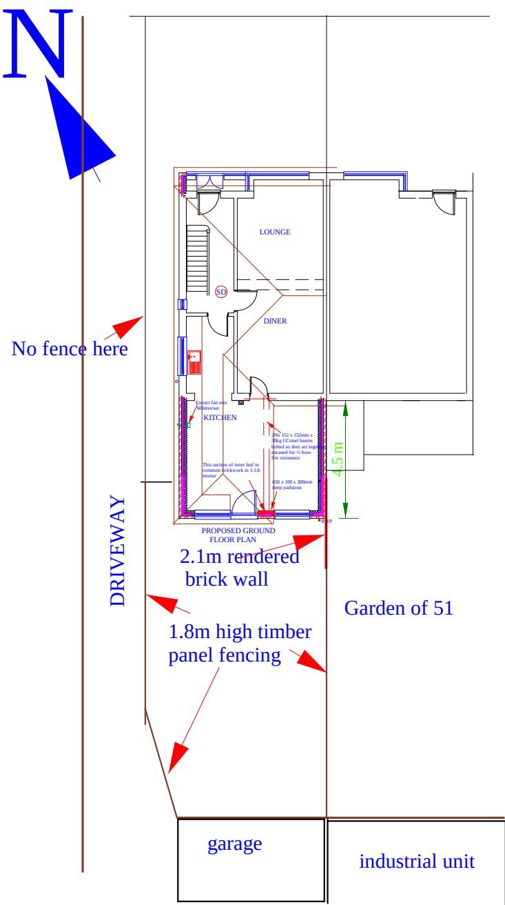
SITE PLAN 1 : 200
