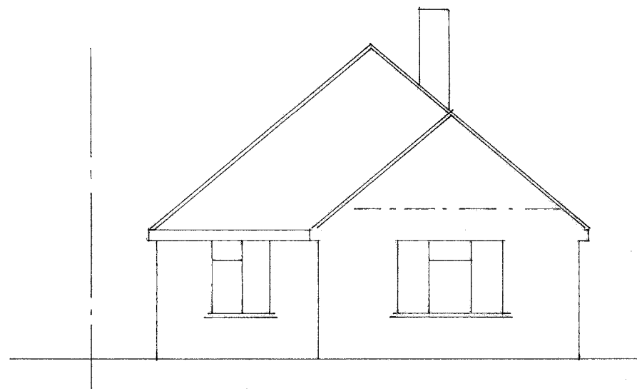
Existing NE/Front Elevation
