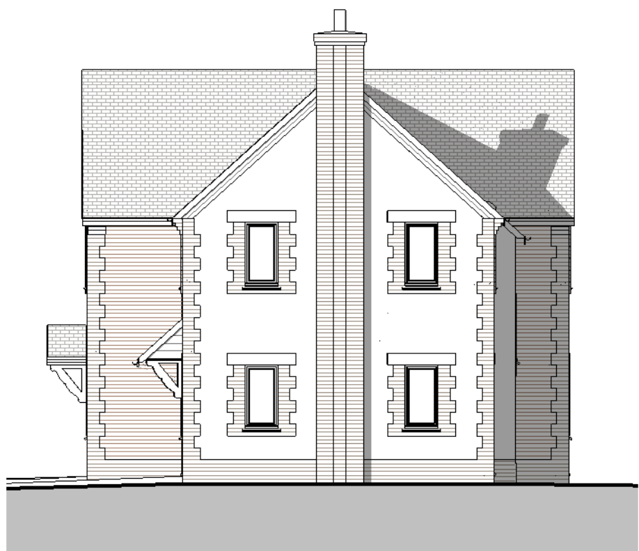
Type 4- Plots 5,6 Right Elevation 1 : 100
