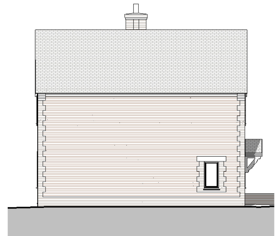
Type 4- Plots 5,6 Left Elevation 1 : 100
