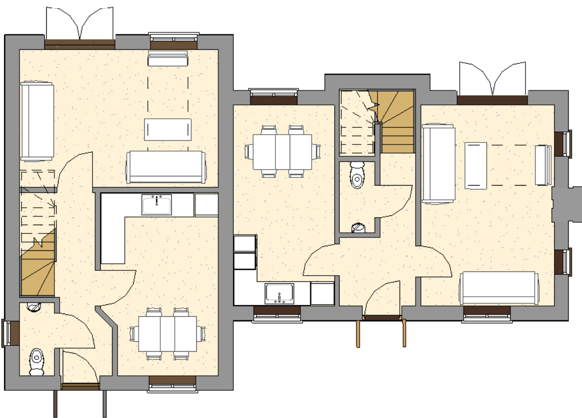
Type 4- Plots 5,6 Ground Floor 1 : 100
