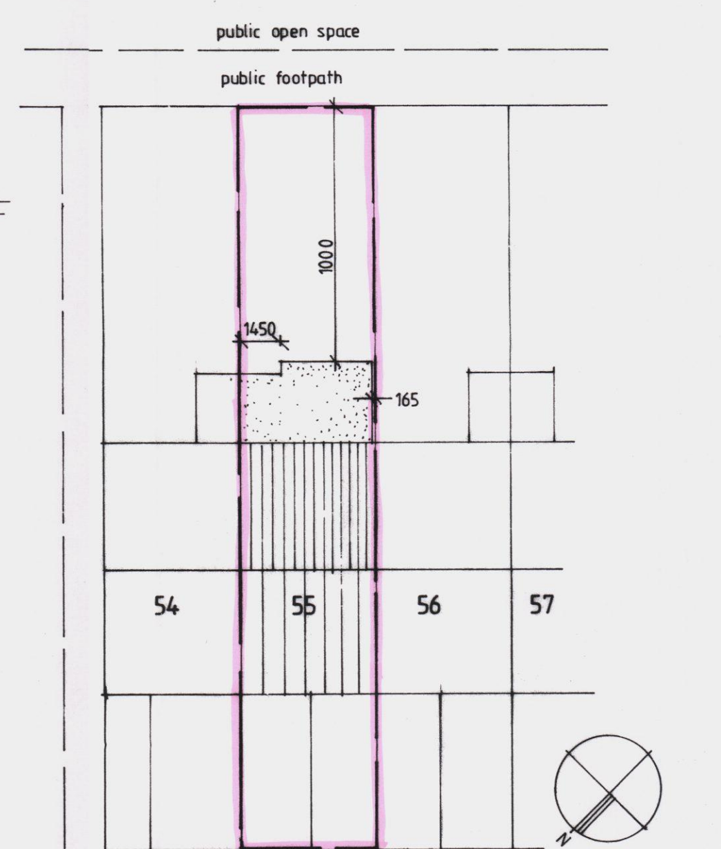
site plan 1/200
