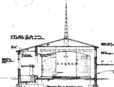
SECTION D-D
