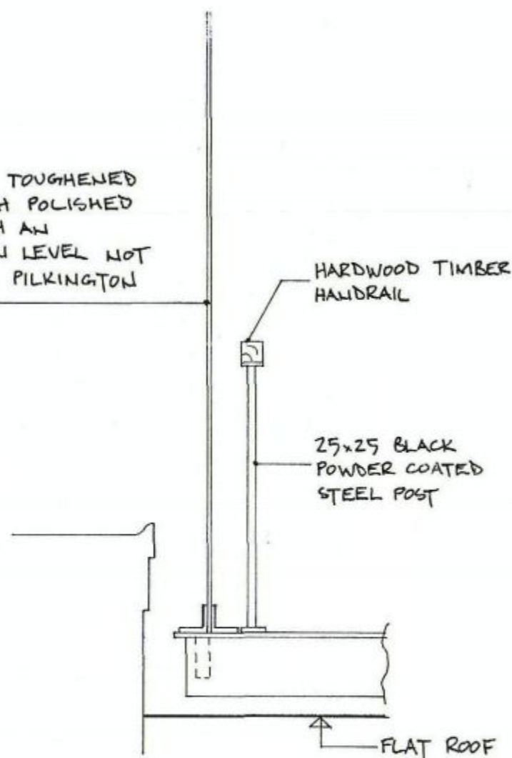
SECTION A-A 1:20
