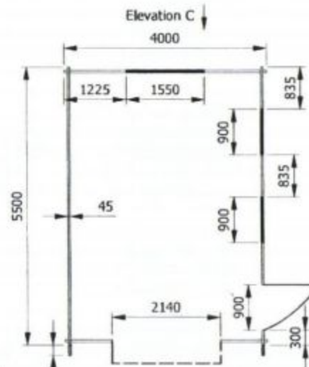
Elevation A
