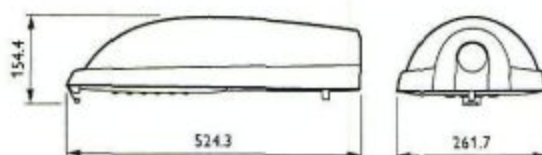
Mini Iridium LED BGS451
