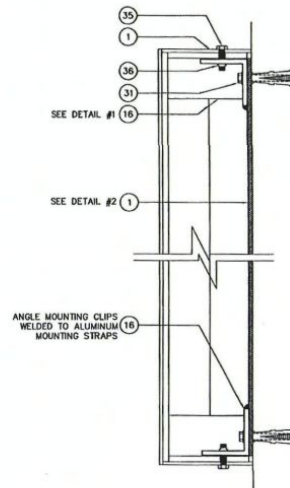
A SECTION SCALE: 3"=1'-0"
