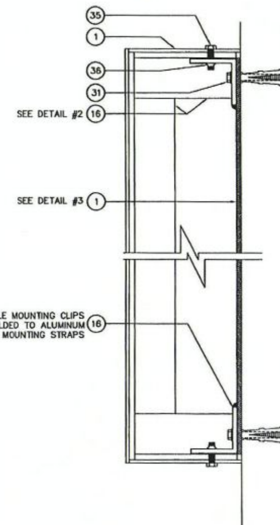
SECTION A SCALE: 3'-1'-0"
