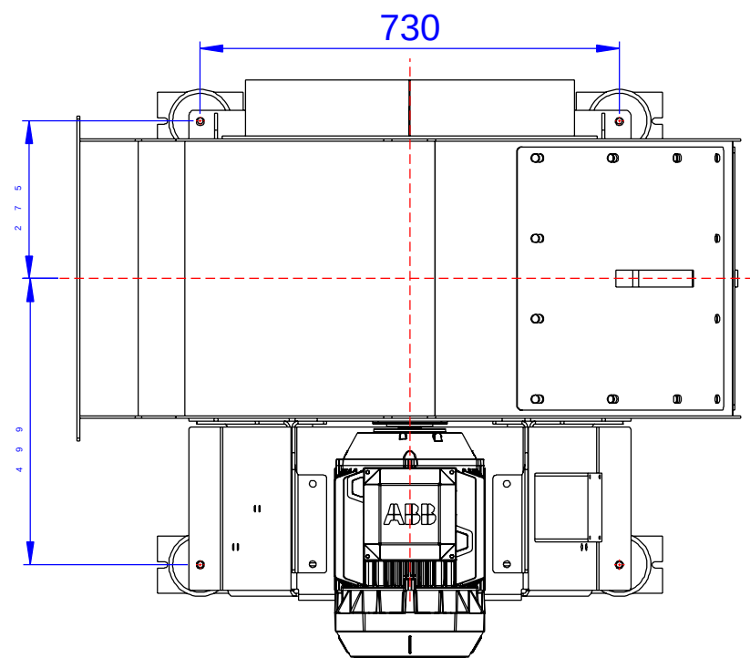
AV MOUNT LOCATION PLAN VIEW
