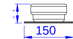
AV MOUNT DETAIL (LSEB TYPE - 4 OFF)
