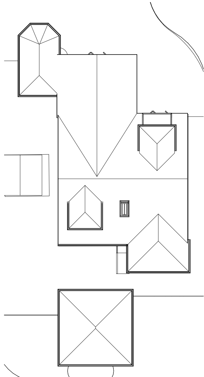
3 Roof Plan 1 : 200
