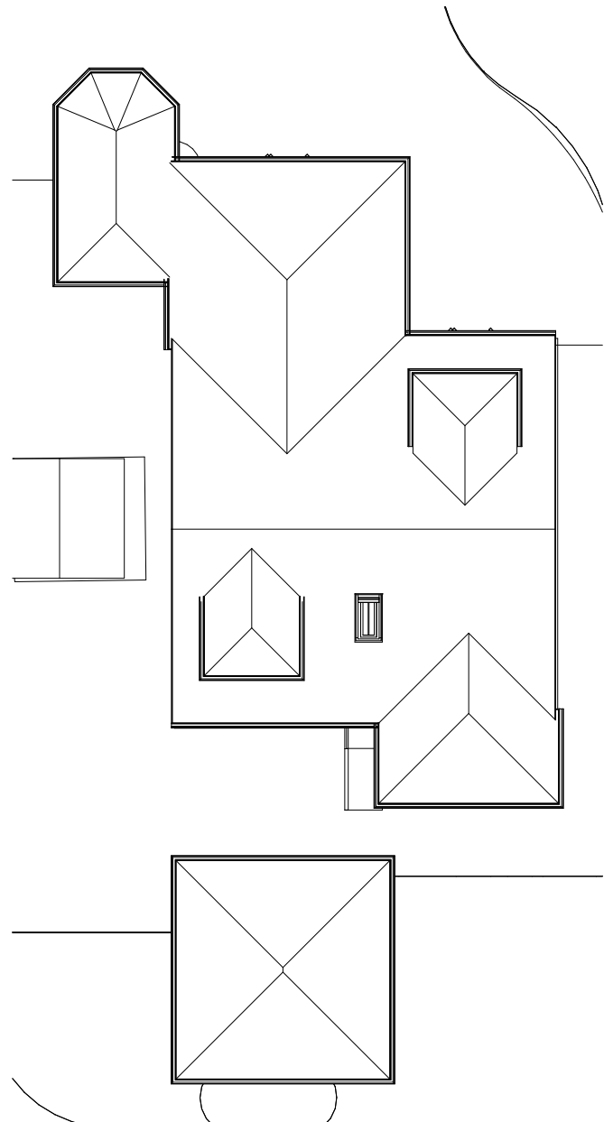
3 Roof Plan 1 : 200
