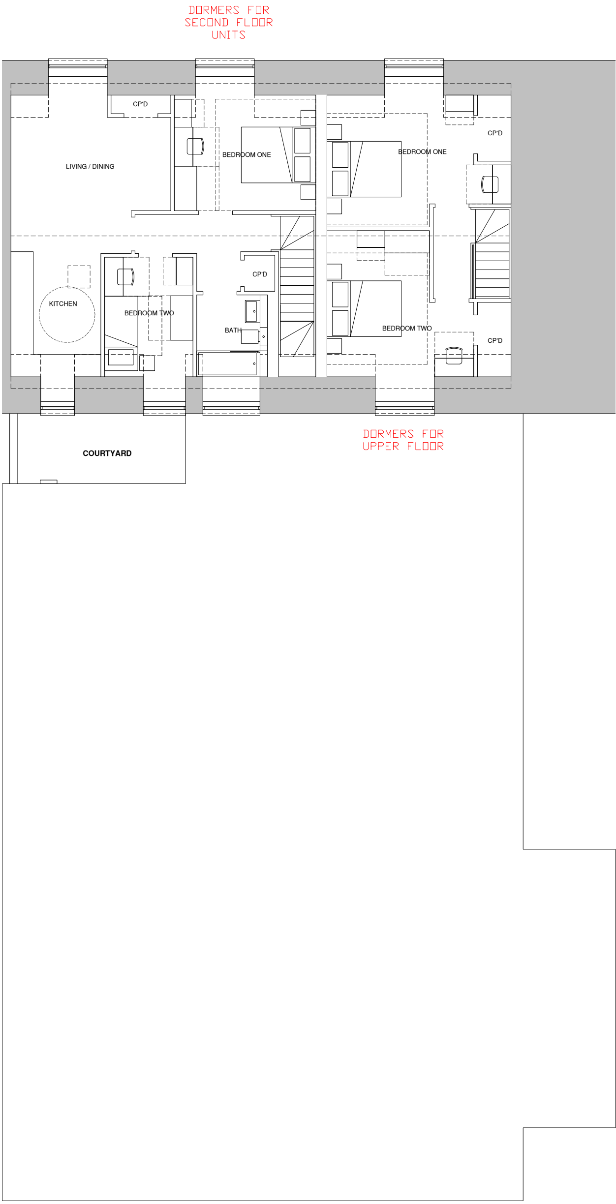
Loft Plan 1:100
