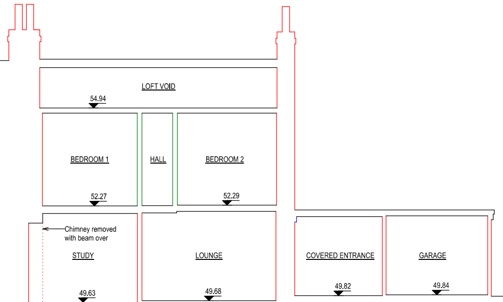
6 EXISTING SECTION A-A Scale: 1:100
