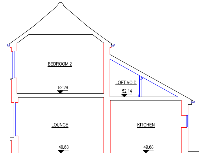
4 EXISTING SECTION B-B Scale: 1:100
