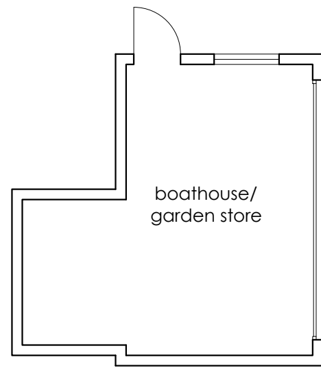
PLAN 1:100
